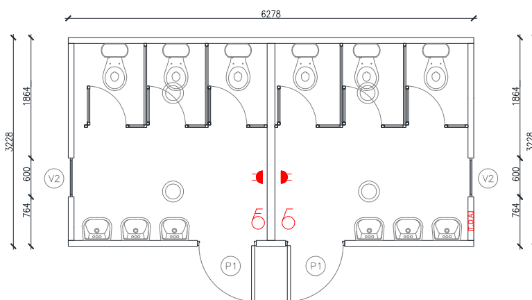
PLANTA REFERENCIAL MOE 20'
