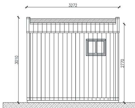
ELEVACIÓN VISTA - A
